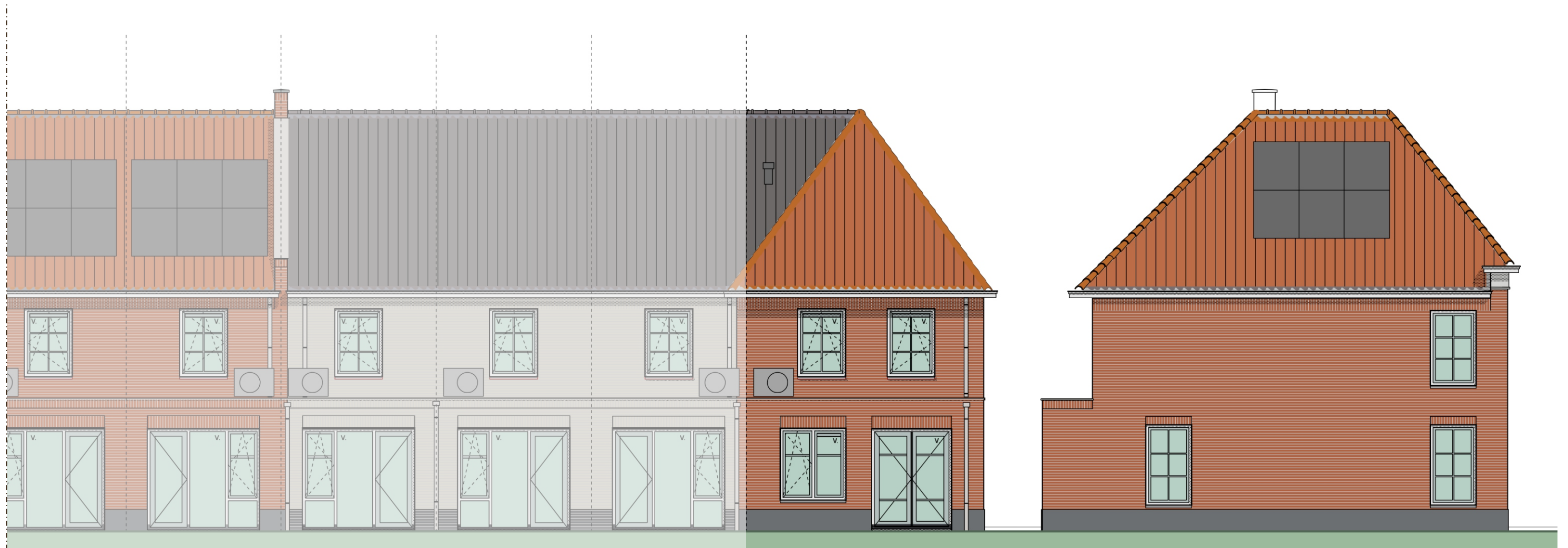
Achtergevel
